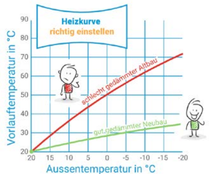
Abbildung 1: Heizkurve (Bildquelle: heizungsmacher.ch)
