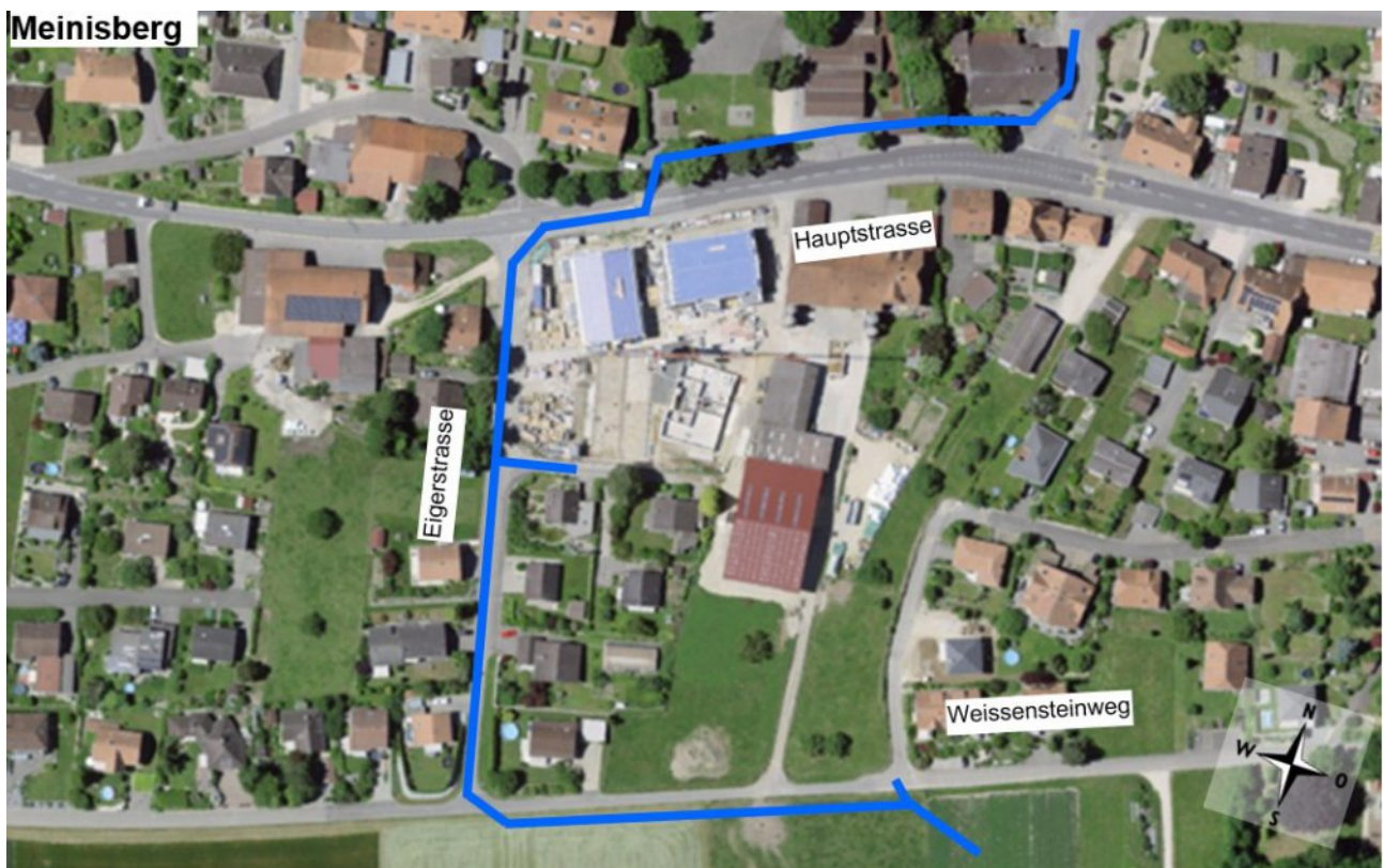
Abbildung 2, Linienführung Regenabwasserkanalisation (Quelle: www.geo.admin.ch )
