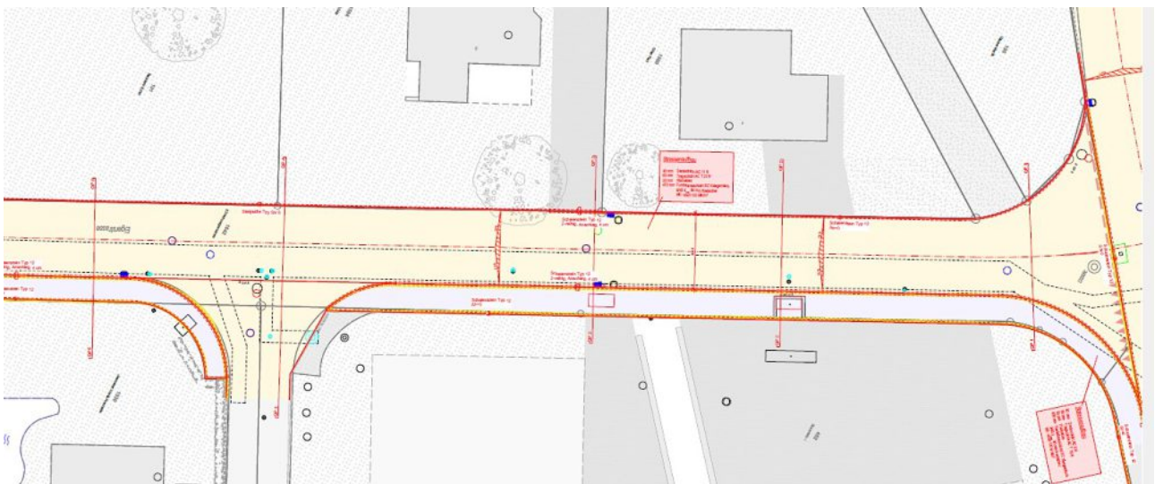
Abbildung 3, Auszug Strassenbauplan Eigerstrasse (Quelle: RSW AG)
